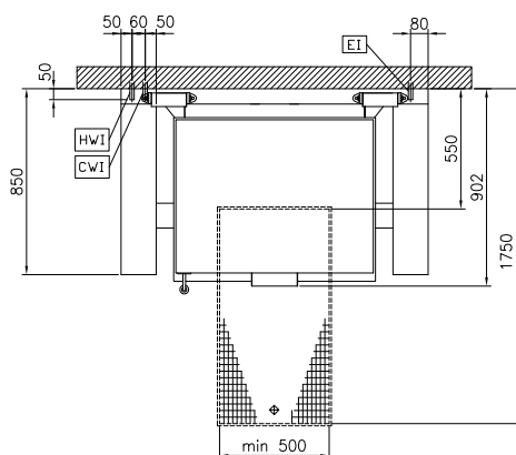
Boven aanzicht
