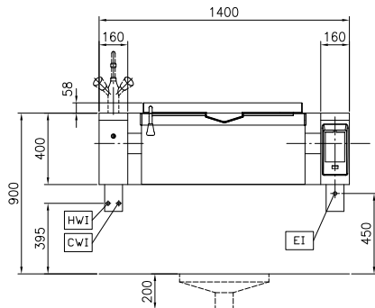
Front aanzicht
